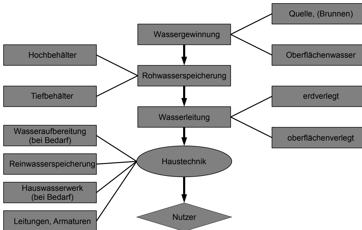
Abbildung 76: Schema Wasserversorgung
