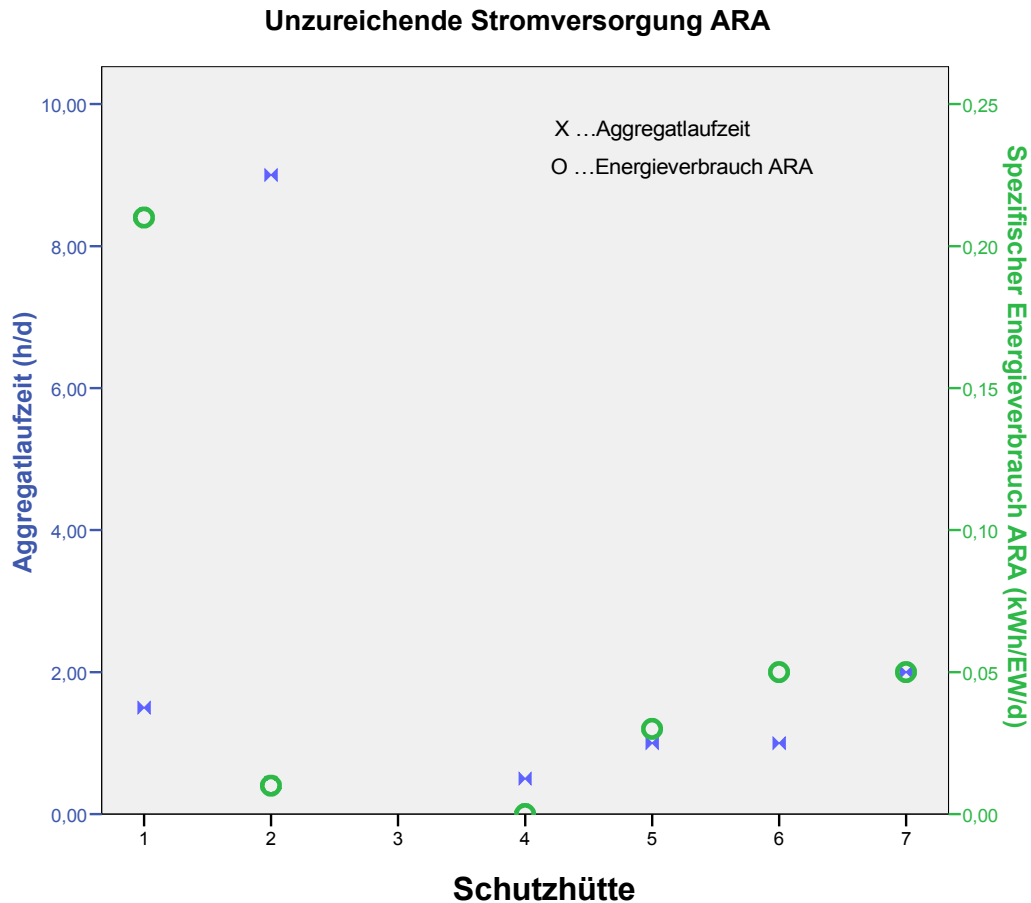
Abbildung 152: Einzelhütten mit Problemen bei der Stromversorgung der ARA (Darstellung der Aggregatlaufzeiten [h/d] und des spezifischen Stromverbrauchs [kWh/EW 60 /d])[58]
