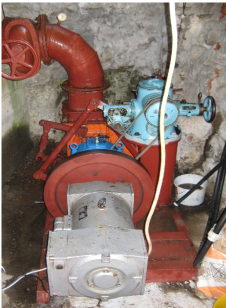
Abbildung 30: Peltonturbine mit 11 kW elektr. Leistung
