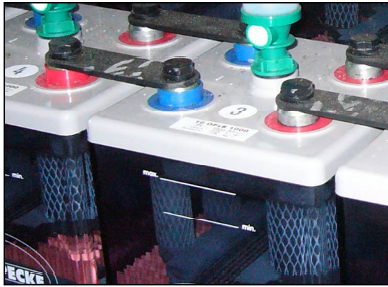
Abbildung 36: Blei-Flüssig-Batterie
