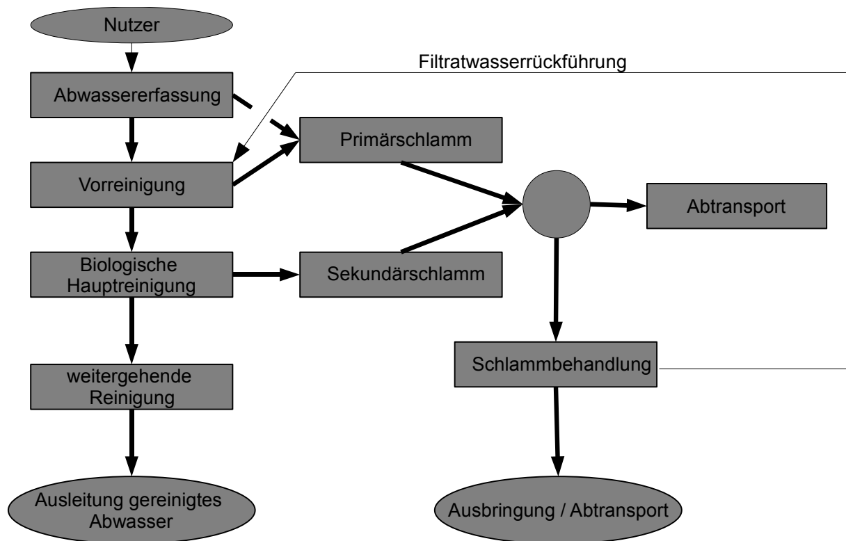
Abbildung 98: Schema Abwasserreinigung
