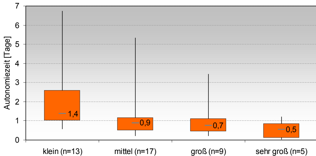
Abbildung 66: Autonomiezeit der Stromversorgung in Bezug zur Hüttengröße
