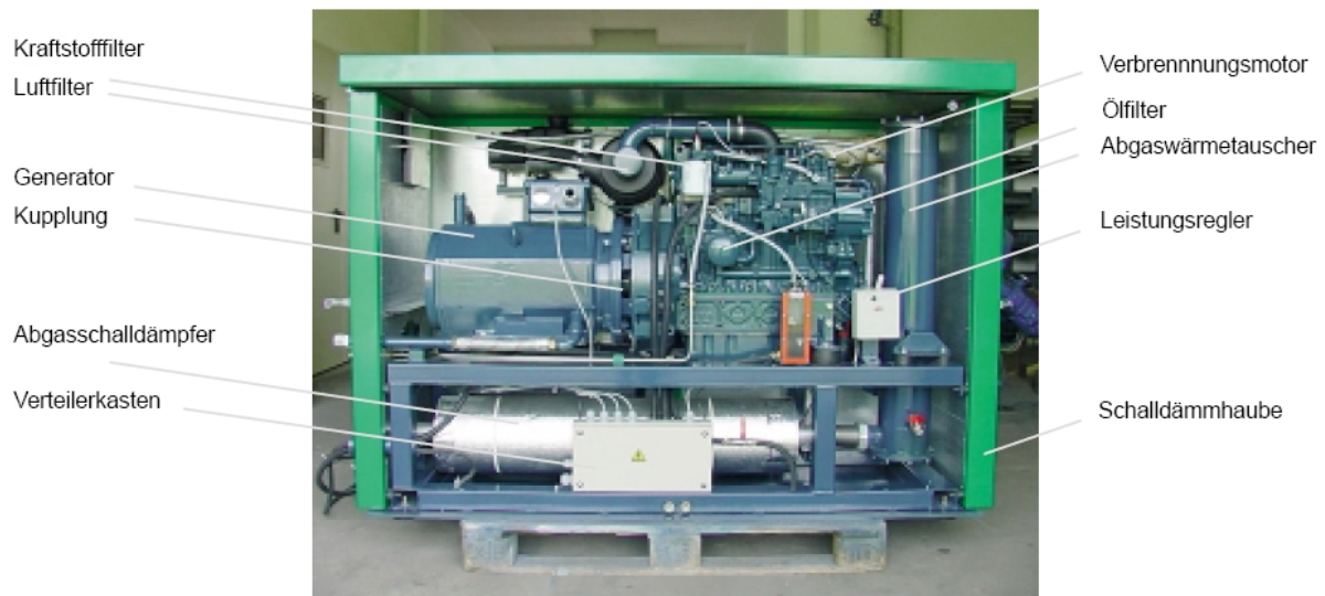
Abbildung 26: Aufbau und Bestandteile eines BHKW [55]
