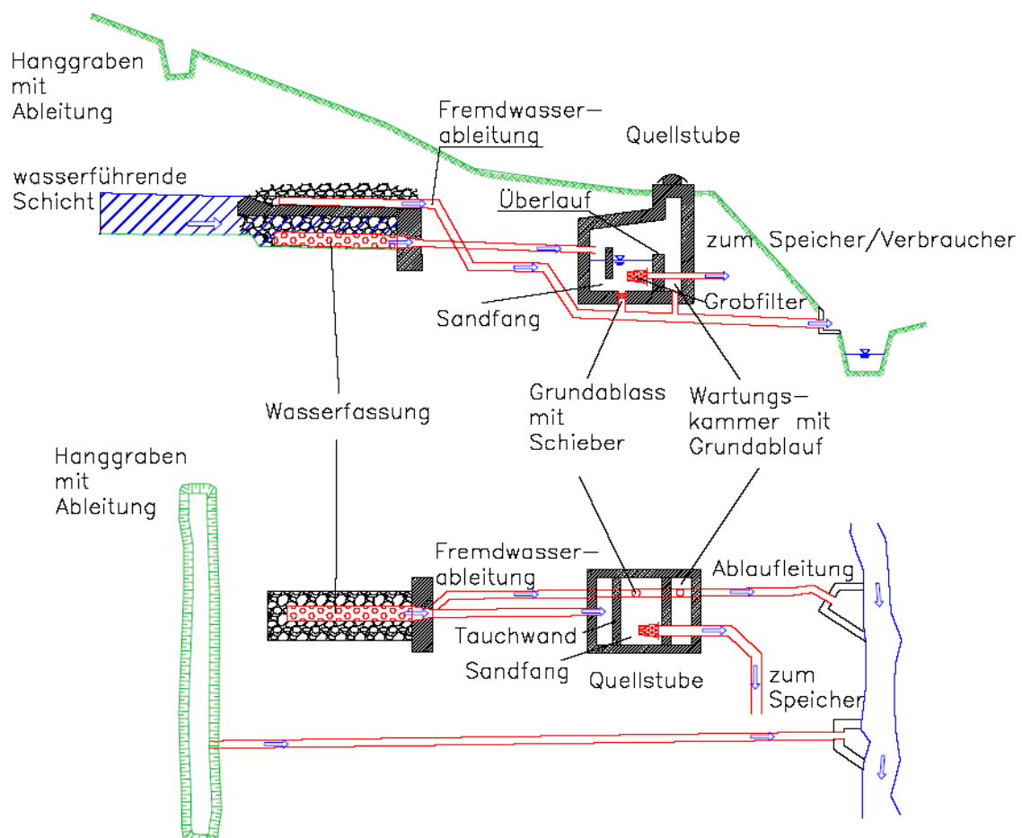
Abbildung 78: Schema Quellversorgung
