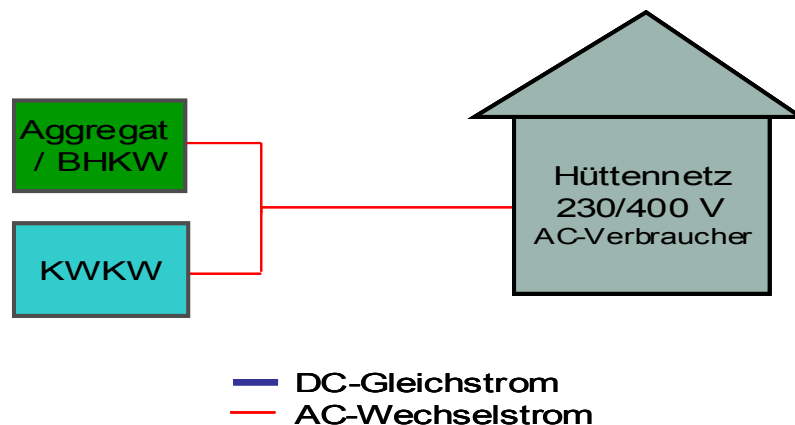
Abbildung 44: Direkte AC-Kopplung der Stromerzeuger mit den Verbrauchern im reinen Wechselstromsystem
